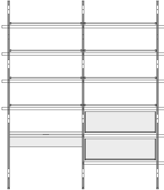
Comp. 301 224,1 x 63 x H 260 cm 3xM2 + 8xR2 + 1xS1 + 2xC3
