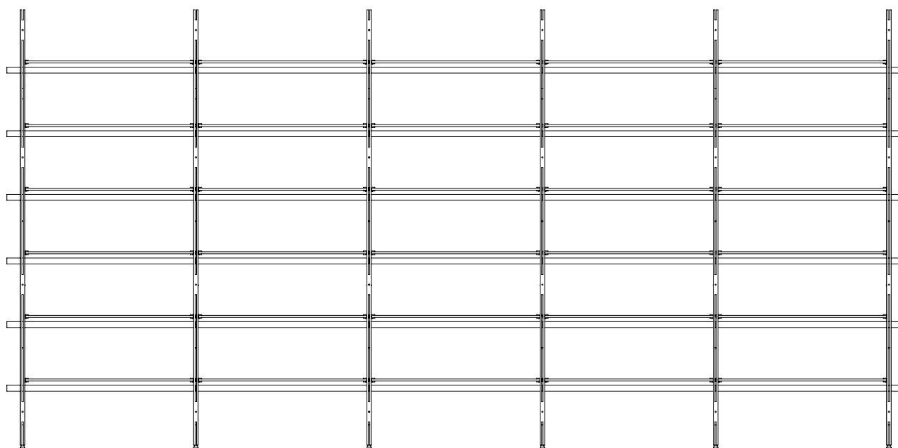
Comp. 603 532,2 x 37 x H 260 cm 6xM2 + 30xR2
