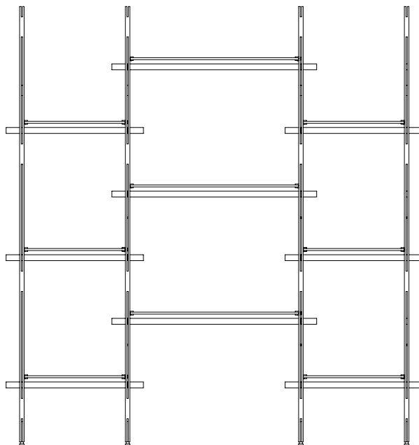
Comp. 409 246,8 x 37 x H 260 cm 4xM2 + 6xR1 + 3xR2
